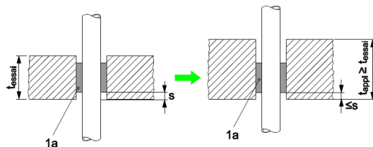
A – Dispositif d’obturation de tuyau entièrement dans un plancher : situation d’essai (à gauche), application pratique (à droite)
